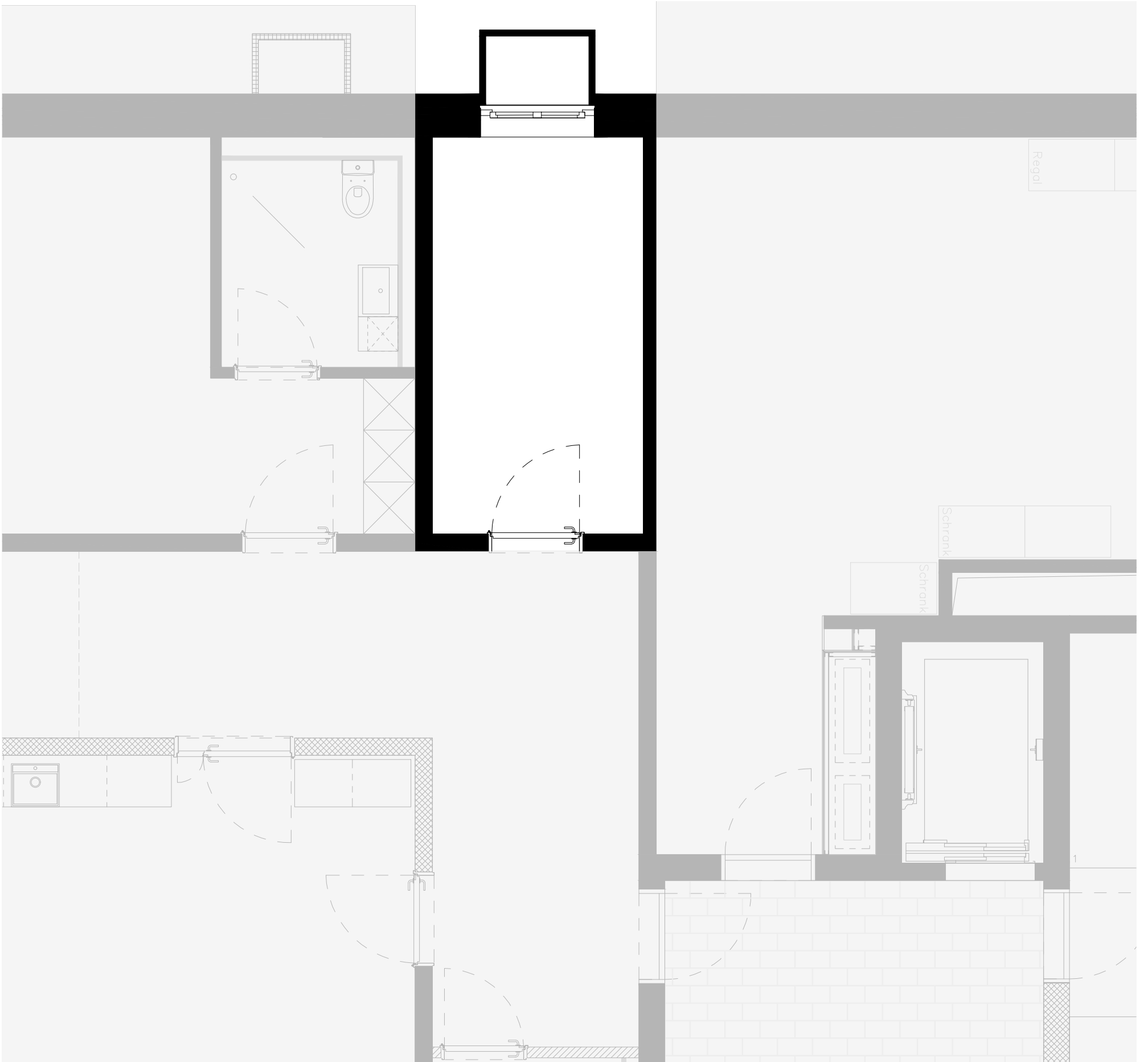
Grundriss, Erdgeschoss M 1:50
