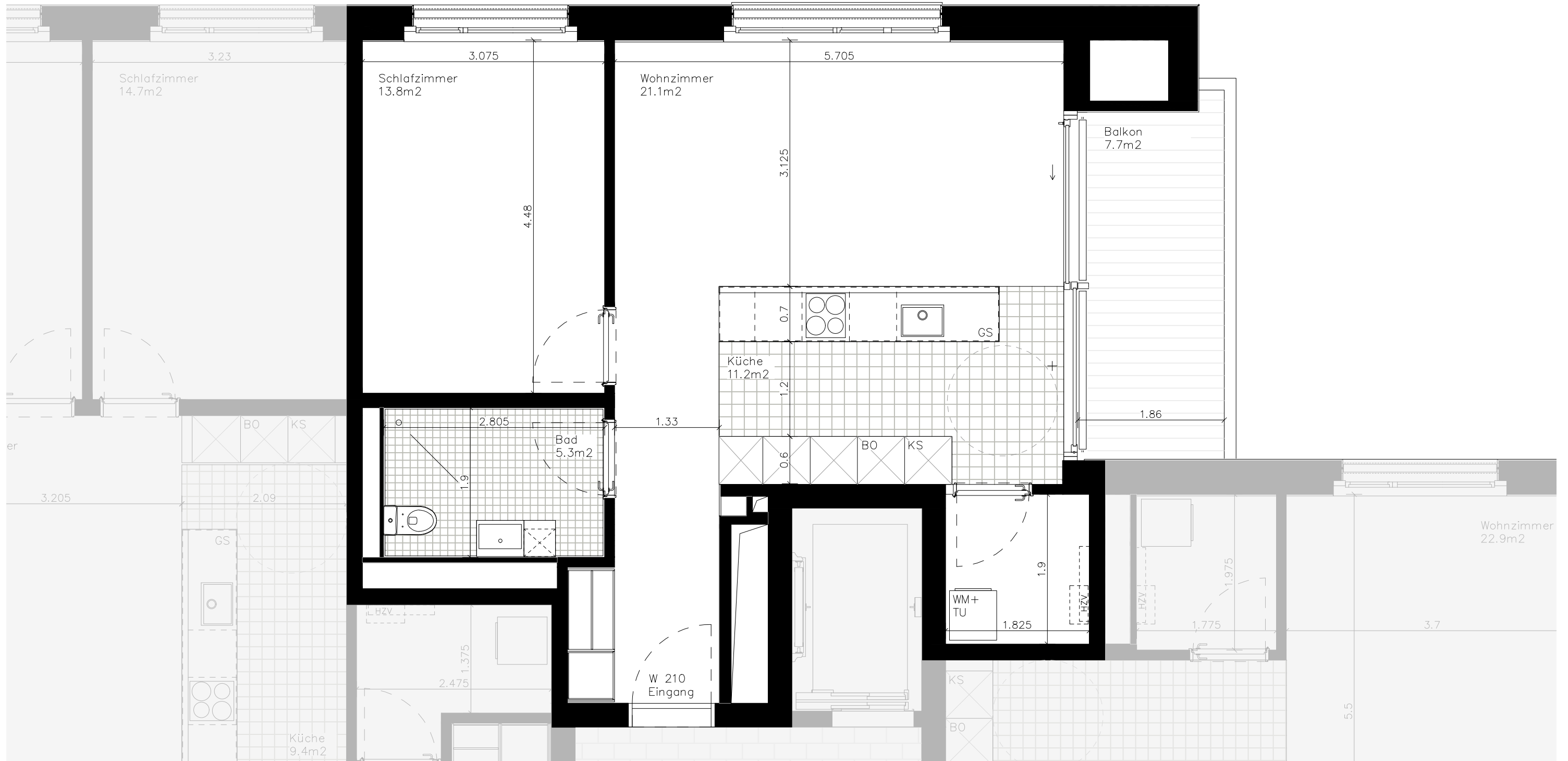
Grundriss, 2.Obergeschoss M 1:50
